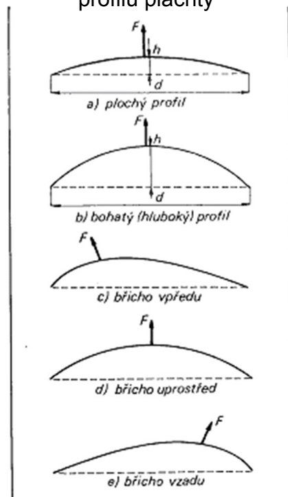
Různé tvary profilu plachty.
